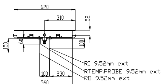
Zij aanzicht
